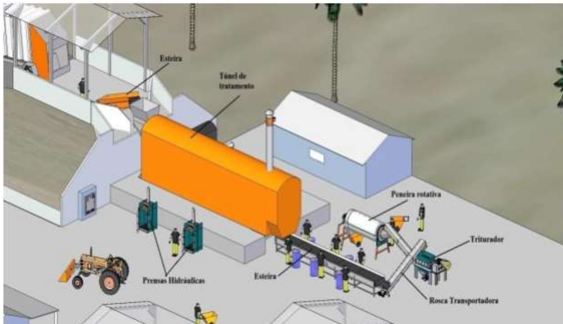
Figura 10: Infraestrutura de uma Central de Triagem e Compostagem
