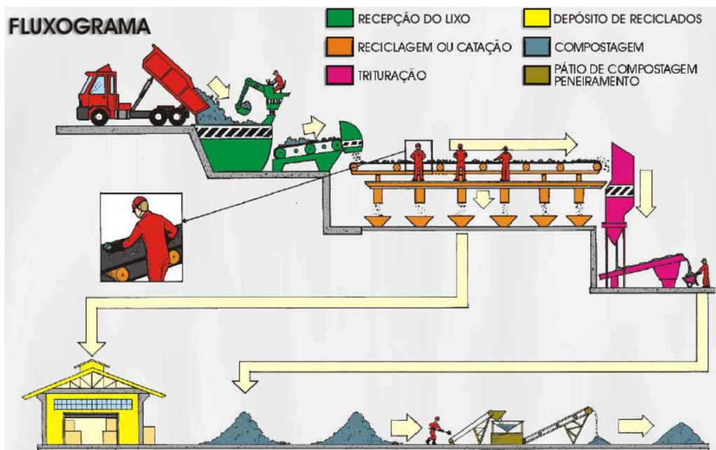
Figura 9: Fluxograma de Processos Usina de Triagem e Compostagem Outra opção indicamos também a Central Modelo Umutorno. Conforme figura abaixo.
