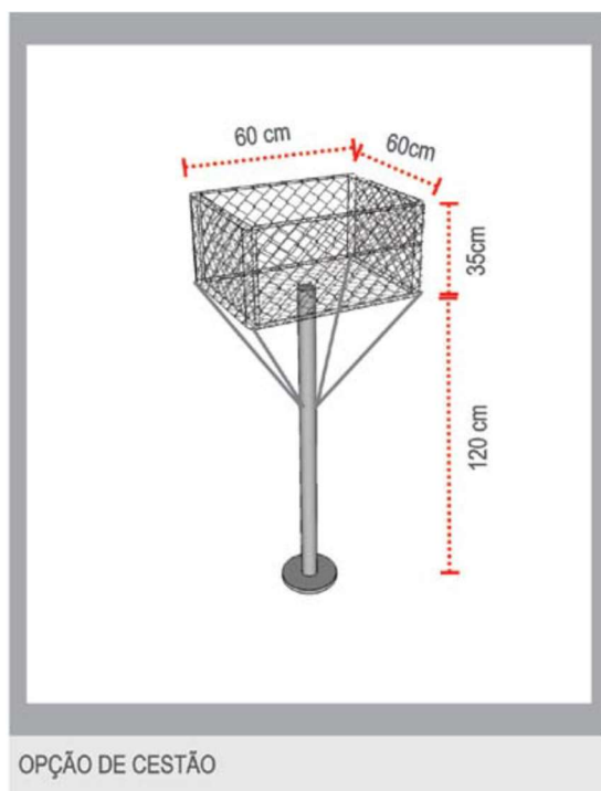
Figura 7: Exemplo de cestão individual
