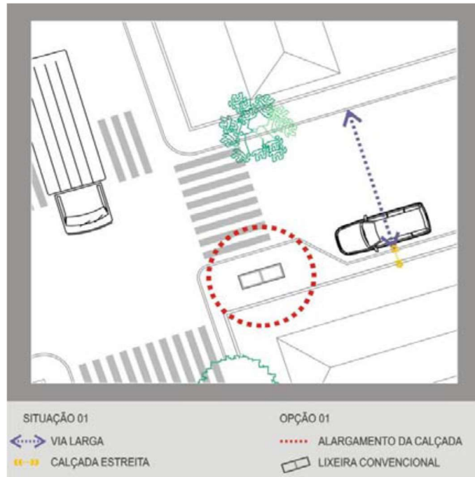
Figura 3: Implantação de cestos comunitários em situações de ruas largas e calçadas estreitas. Fonte: ProResíduos/UEM, 2020
