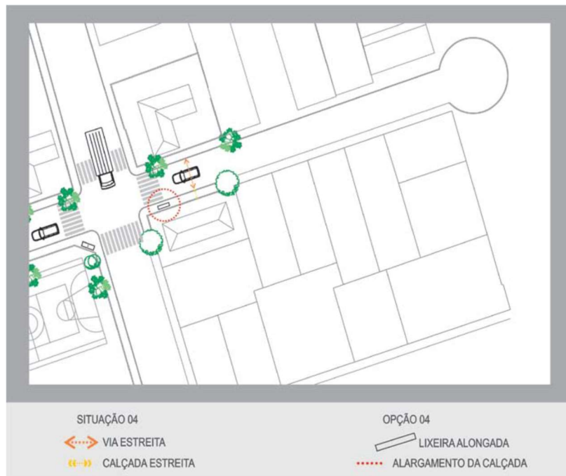
Figura 6: Implantação de cestos comunitários em situações de vias e calçadas estreitas e sem saída. Fonte: ProResíduos/UEM, 2020
