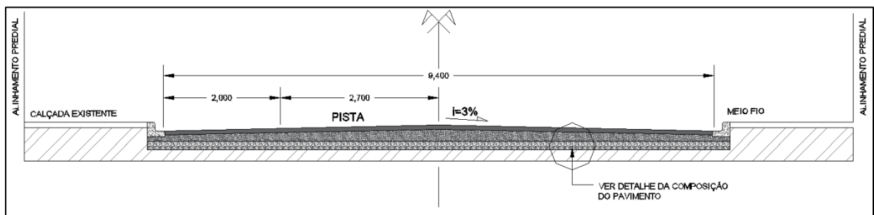
Figura 2 – Seção transversal
