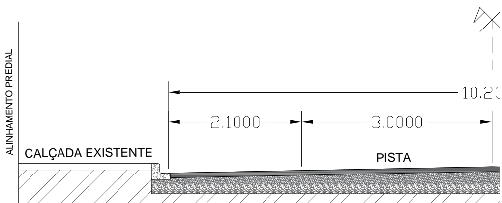
Figura 3 – Meia Seção transversal
