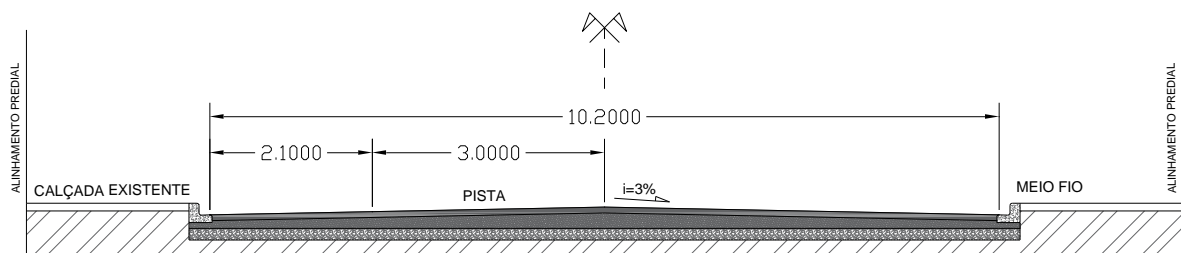
Figura 2 – Seção transversal
