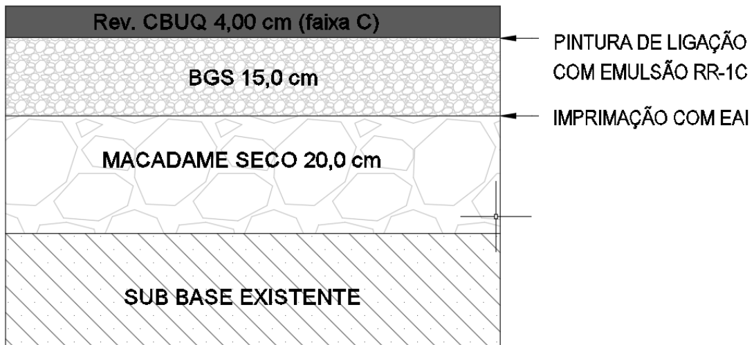
Figura 15 – Camadas finais de projeto
