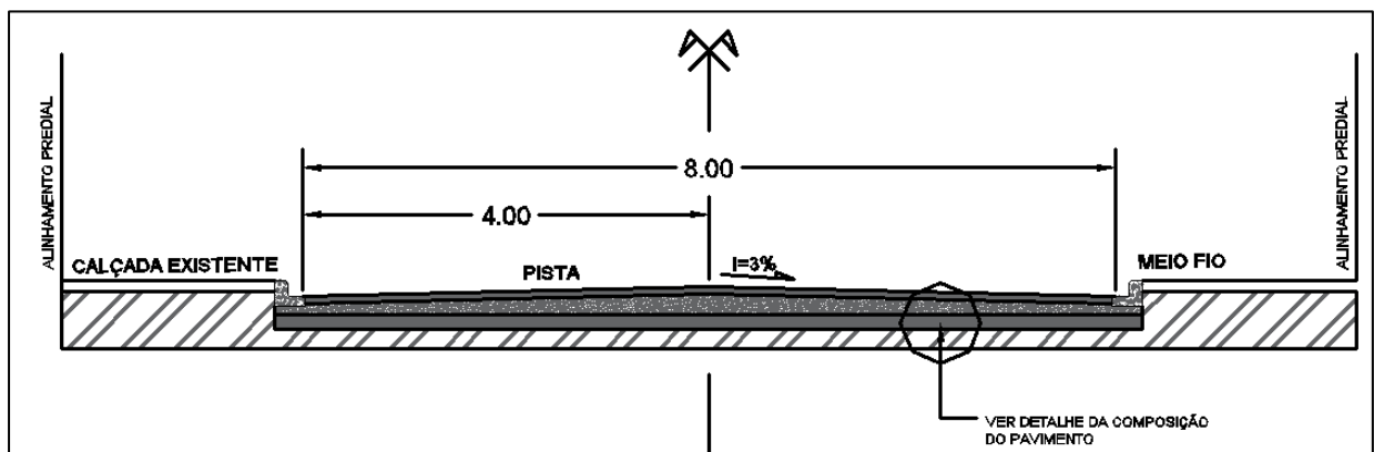
Figura 2 – Seção transversal
