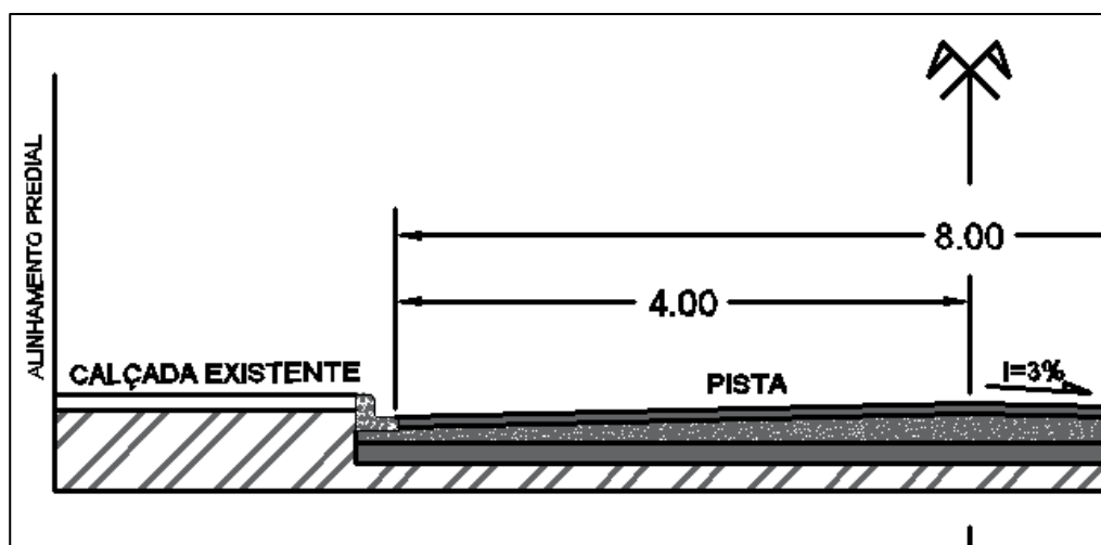
Figura 3 – Meia Seção transversal
