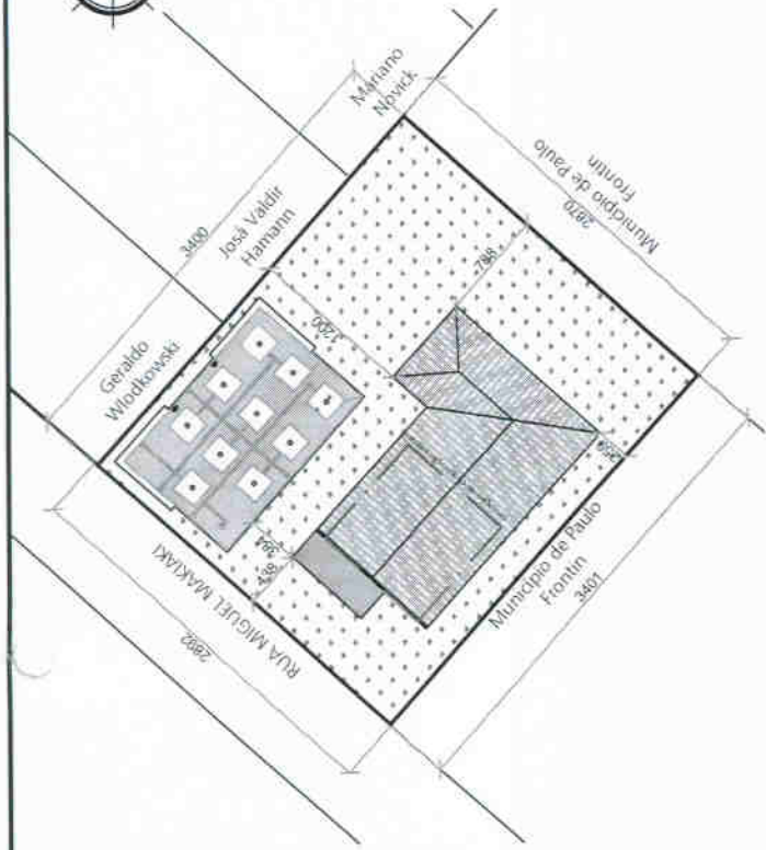
01 IMPLANTAÇÃO Escala 1:2,00
